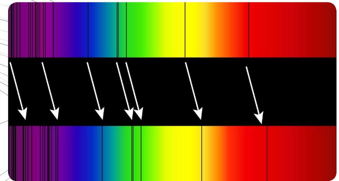
Προσομοίωση της μετατόπισης προς το ερυθρό του γαλαξιακού υπερσμήνου Bass 11 (κάτω), σε σχέση με το φάσμα του Ήλιου (πάνω).
